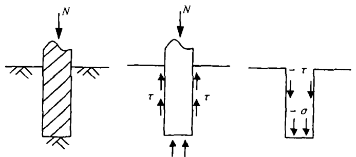
(a)嵌岩桩的嵌岩段 (b)桩的嵌岩段受力 (c)岩体受力分析
