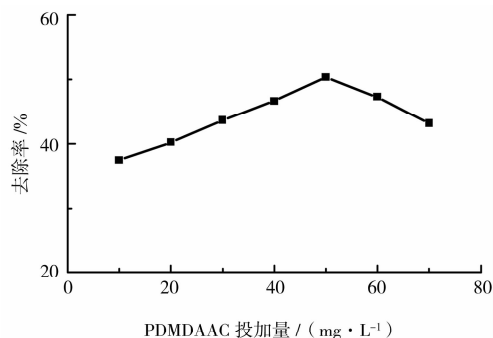
图 1 PDMDAAC 投加量对去除率的影响
