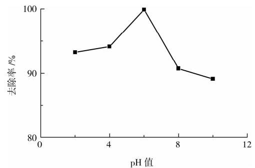
图 3 pH 值对去除率的影响
