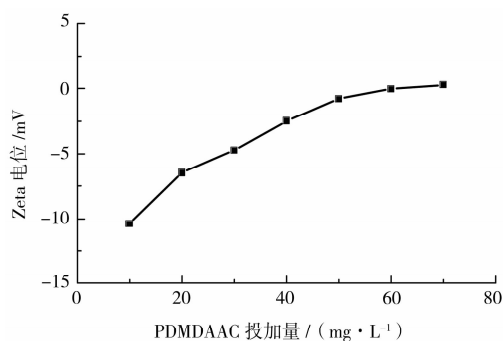
图 5 PDMDAAC 投加量对 Zeta 电位的影响
