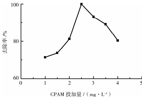
图 2 CPAM 投加量对去除率的影响
