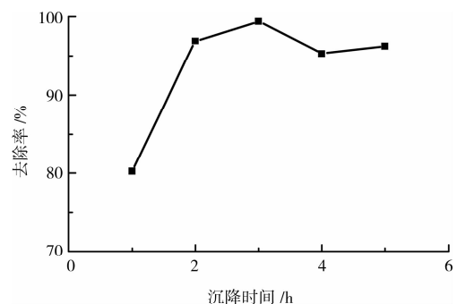
图 4 沉降时间对去除率的影响
