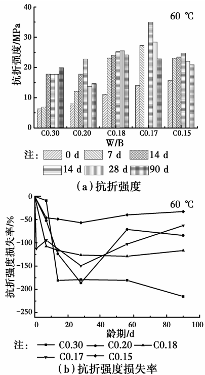
图 4 60 °C 水养护条件下 UHPC 的抗折强度 Fig. 4 Flexural strength of UHPC at 60 °C
