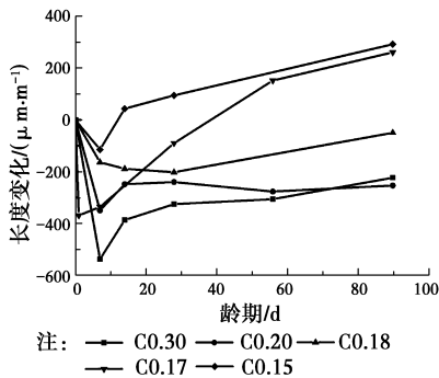
图 3 60 °C 水养护不同水胶比 UHPC 的长度变化 Fig. 3 Influence of W/B on length change at 60 °C
