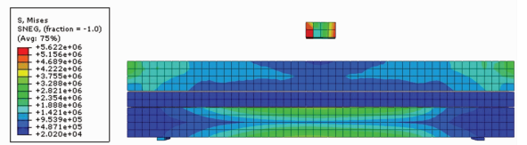
图 12 试件的 Mises 应力分布云图 ( t=20\text{ ms} )
