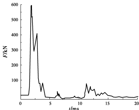
图5 落锤试验冲击力时程曲线
