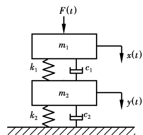
图 2 双自由度弹簧阻尼冲击加载分析模型 Fig. 2 Two-DOF-Spring-Mass-Dashpot impact loading analytical model
