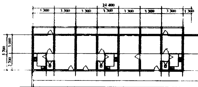
图3 改造后平面图
