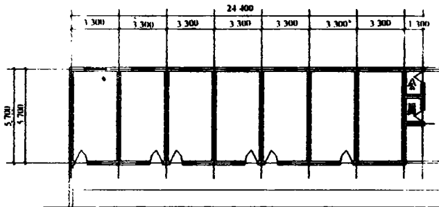
图2 改造前平面图
