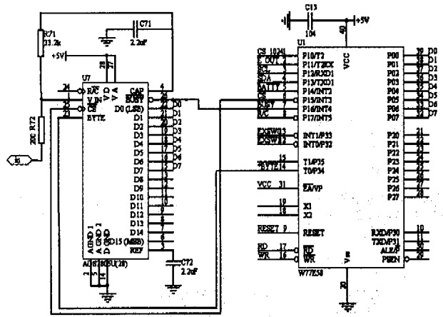
图2 A/D与单片机接口电路原理图
