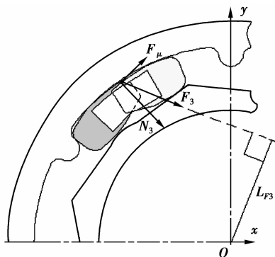
图7 弹簧座楔入接触
