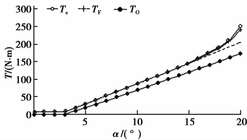
图 13 转矩特性曲线
