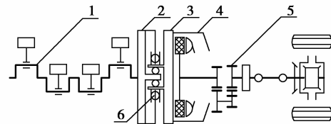
1. 发动机;2. 初级飞轮;3. 次级飞轮; 4. 离合器;5. 变速箱;6. 减振器
