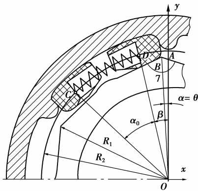
图 4 结构参数坐标系
