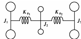
图 14 扭振分析模型
