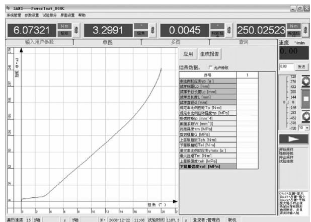
图 12 转矩试验曲线
