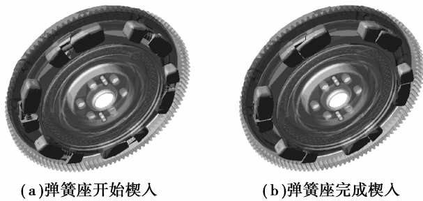
图 9 双质量飞轮加载过程中弹簧座的楔入
