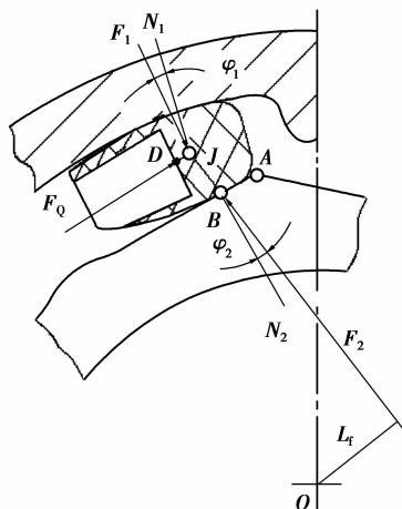
图 5 弹簧座受力分析
