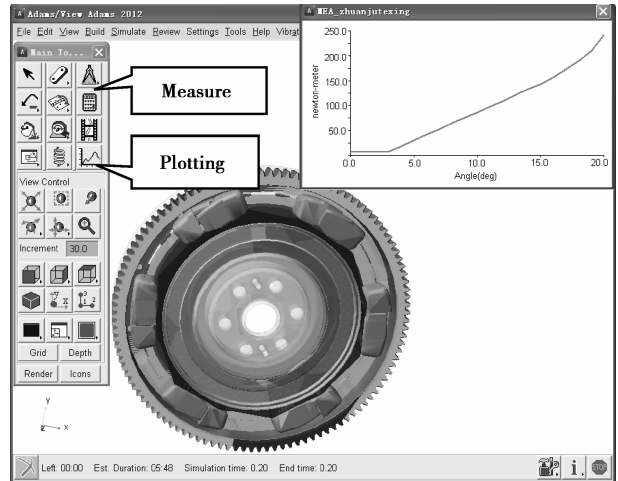
图 10 仿真转矩特性曲线
