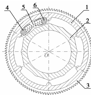
1. 初级飞轮;2. 次级飞轮;3. 启动齿圈; 4. 弹簧座;5. 弹簧
