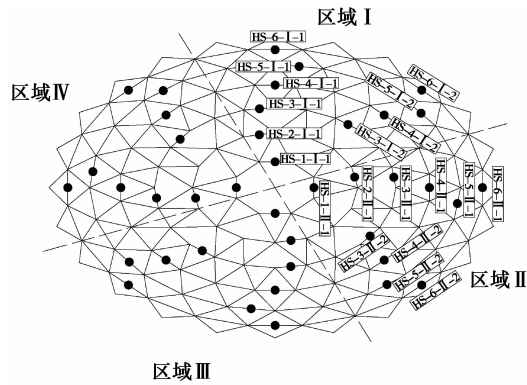
图 4 常州体育馆预应力拉索施工分区及张拉点布置
