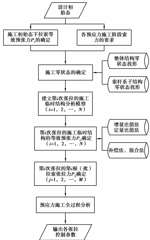
图 2 基于等效预张力的预应力施工过程正算法
