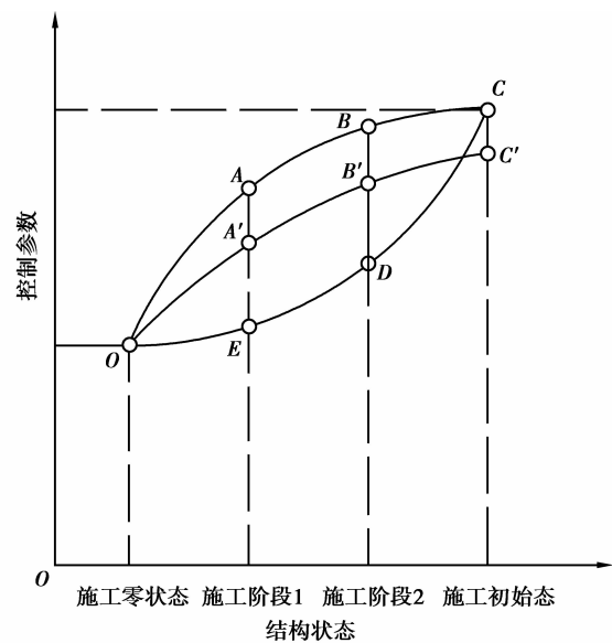
图1 弦支穹顶预应力施工路径图
