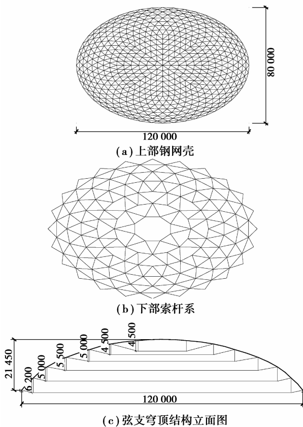
图 3 常州体育馆钢屋盖计算模型简图
