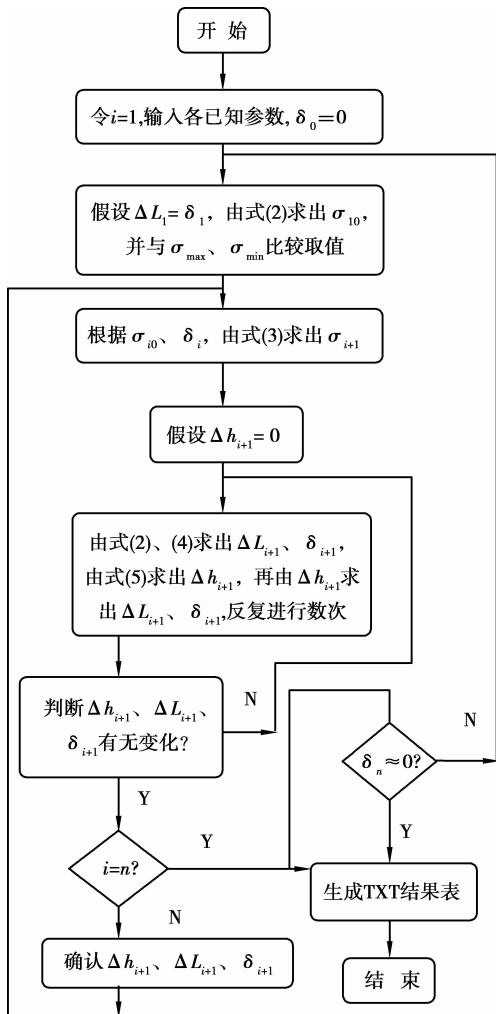
图 3 最大不平衡张力程序设计流程图
