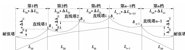
图 1 不均匀覆冰示意图
