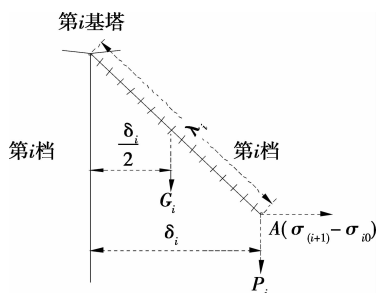
图 2 悬垂绝缘子串受力图
