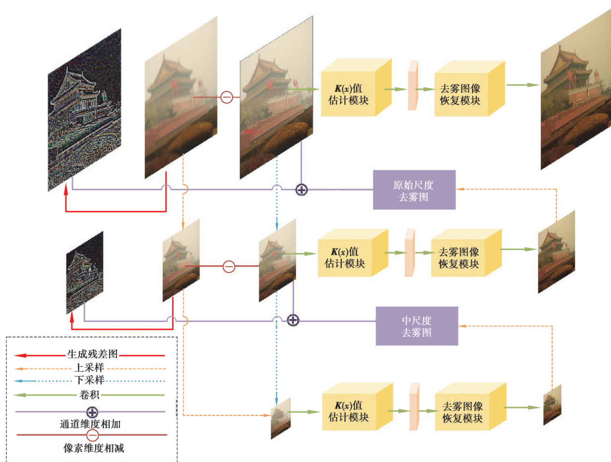
图4 拉普拉斯金字塔型特征提取网络结构
