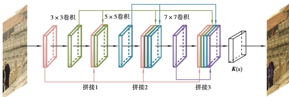
图1 AOD-Net网络结构图
