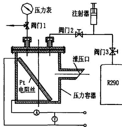
图1 爆炸性试验装置简图
