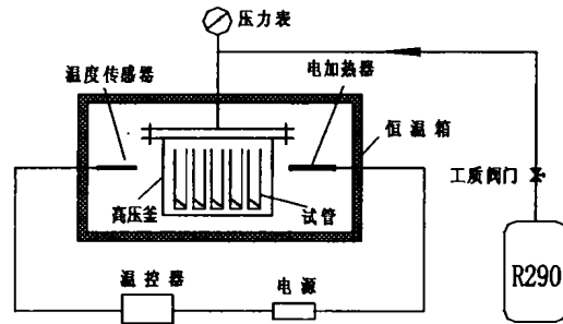
图 3 相容性能试验装置
