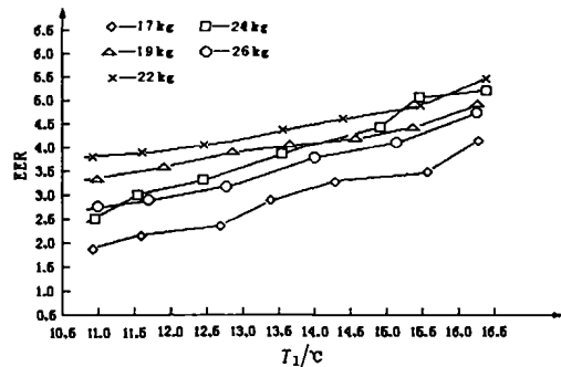
图 6 不同充灌量下 EER 随 T_1 的变化
