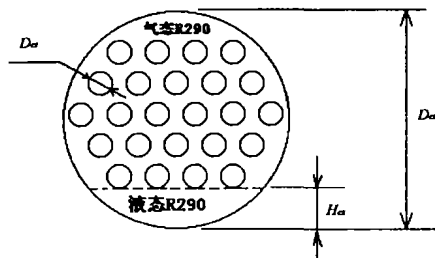
图 4 冷凝器内工质量计算示意图
