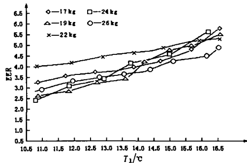
图 7 不同充灌量下 EER 随 T_1 的变化
