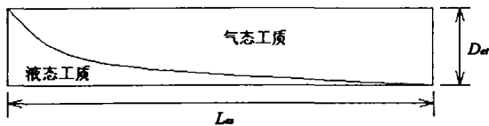
图 5 蒸发器内工质量计算示意图
