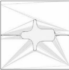
图 4 预锻模拟结果
