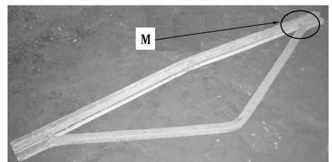
(a) 制动梁架锻件实物照片 缩径
