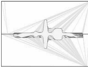
图 5 终锻模拟结果
