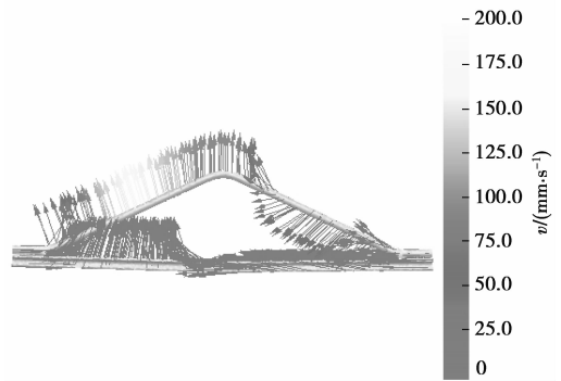
图 7 拉制模拟结束时速度矢量图
