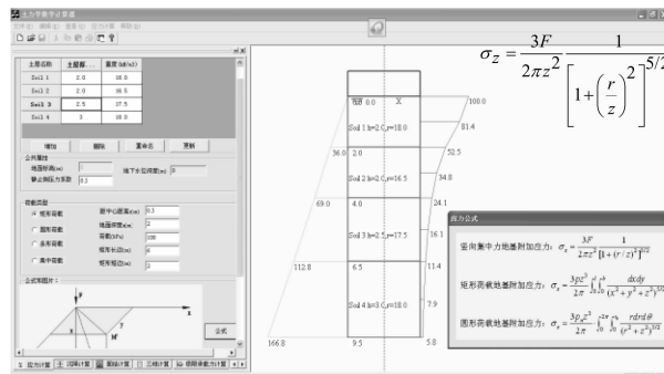
图 1 岩土力学求解器——地基应力计算
